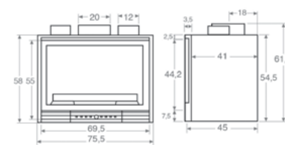
Cristal derecho E055-D
