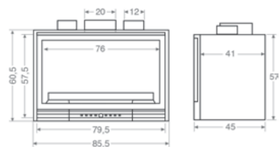
Cristal derecho E063-D
